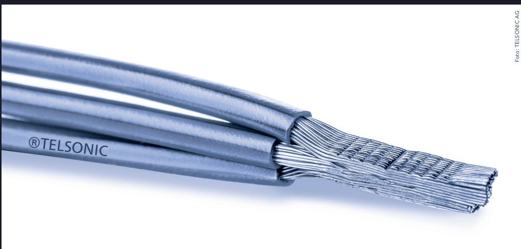
Kompaktieren von Aderenden
